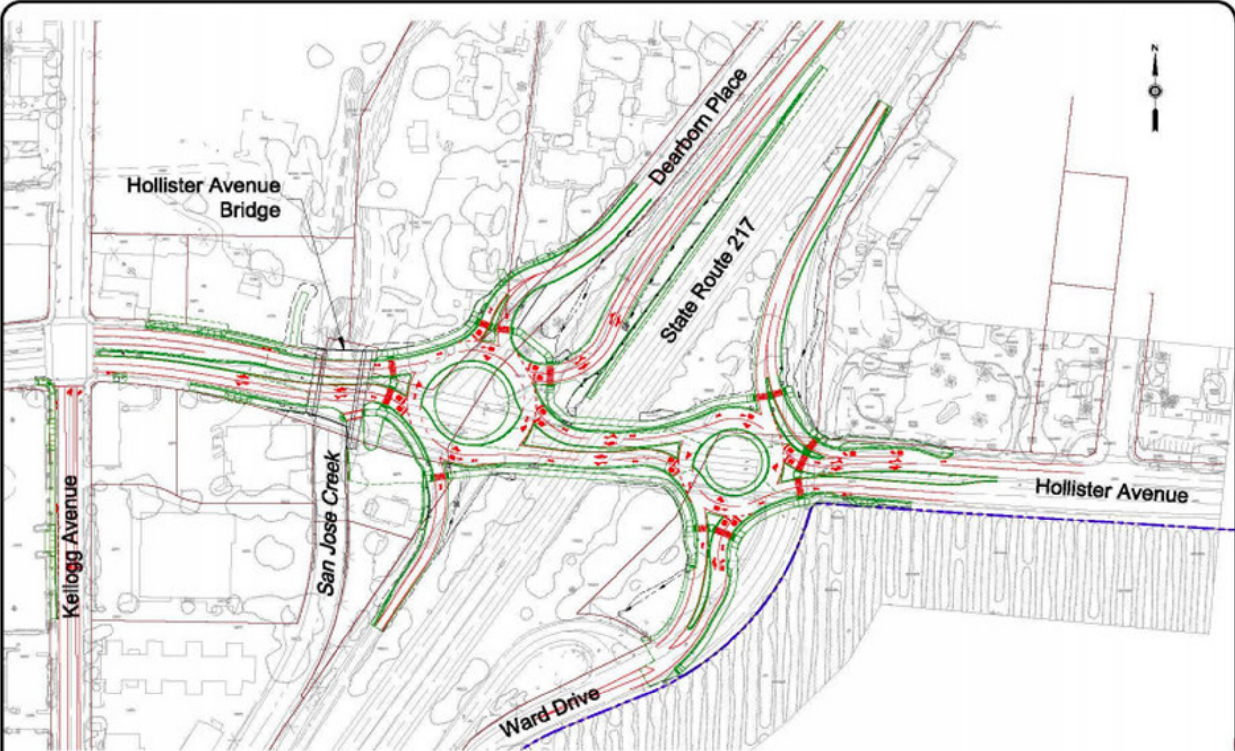
PLAN SCALE: 1"=125'
